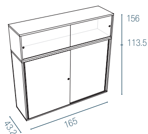
2 portes coulissantes mélamine Réhausse 2 portes Altuglas®
