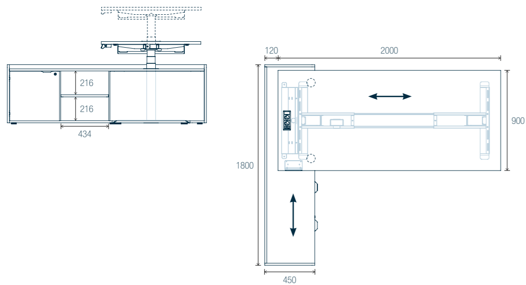
Zicht A - Versie 2 open vakken
