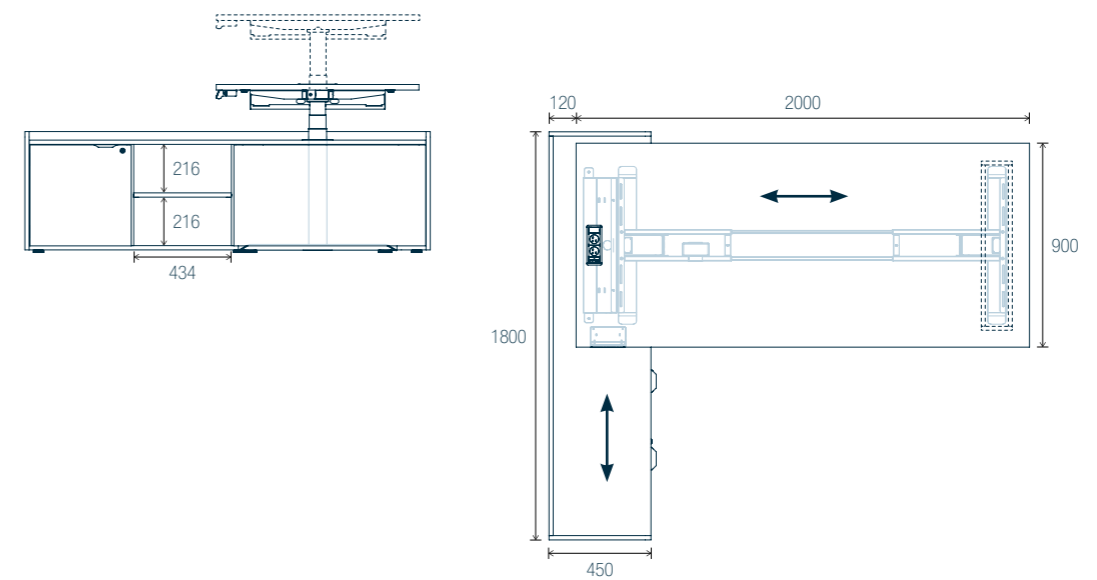
Zicht A - Versie 2 open vakken
