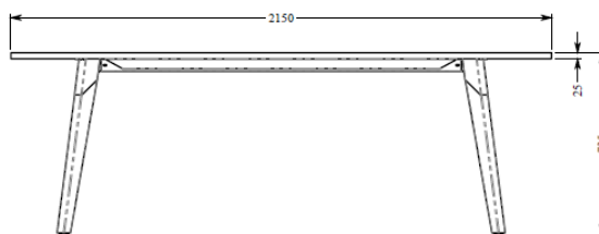
Vooranzicht
