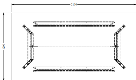
Bovenaanzicht
